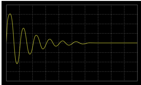
ARB13 2次インパルス応答(減衰係数 0.2)
